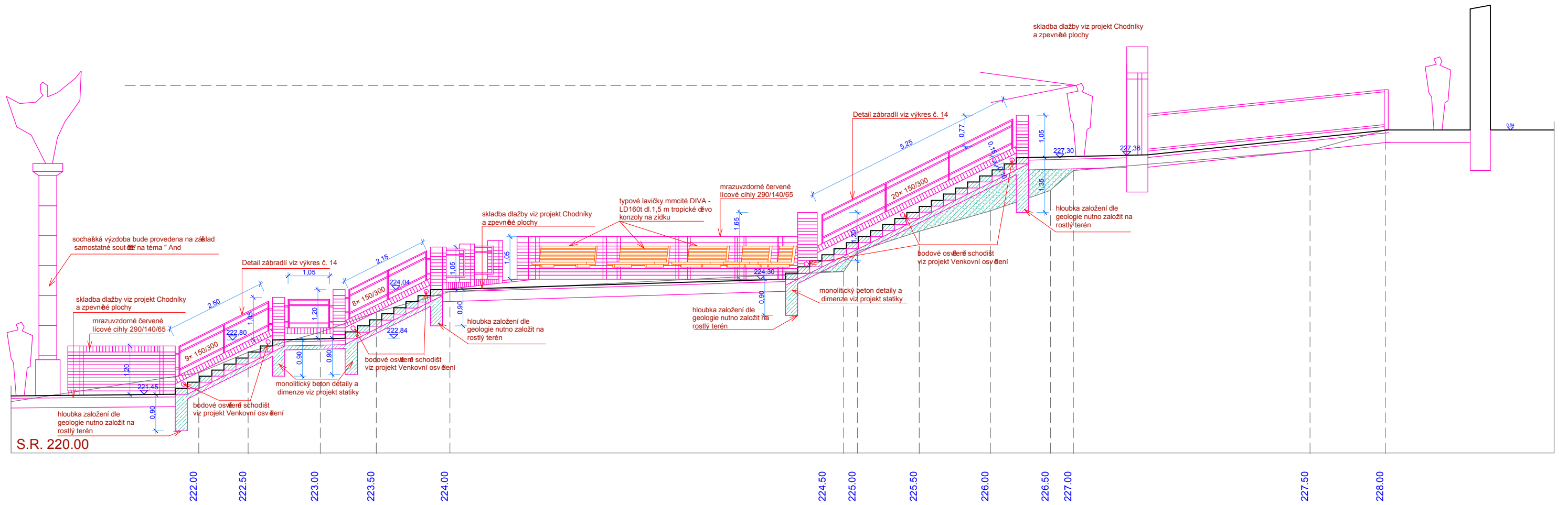
PŘČNÝŘZ AA 1: 200
